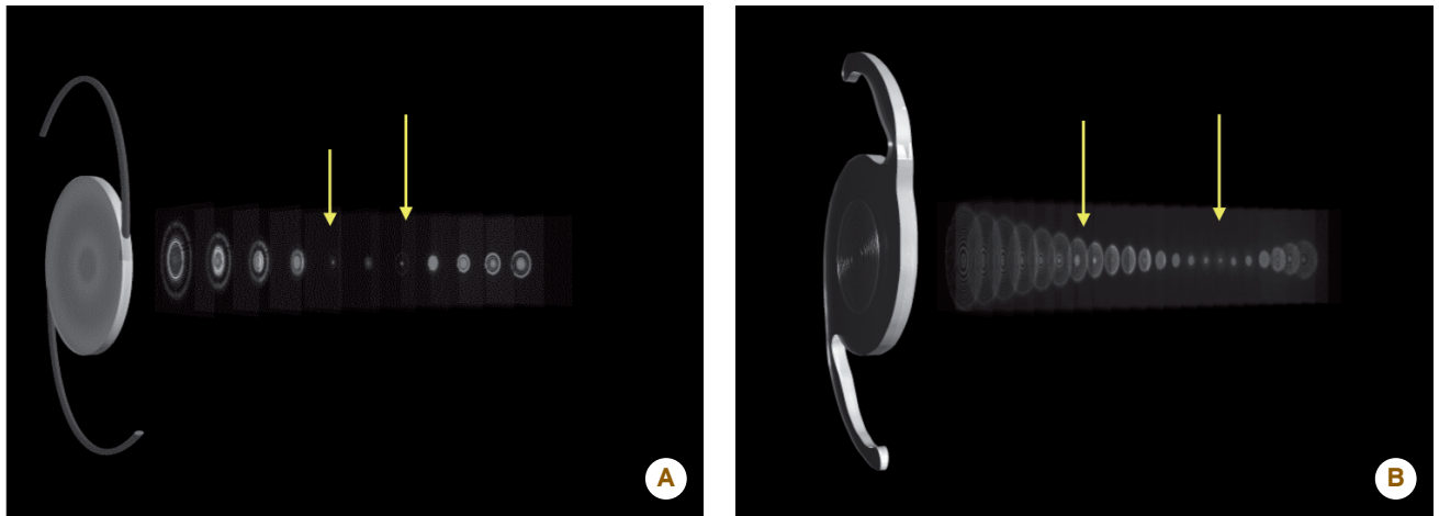
Figure 3 A) Implant réfractif multifocal (ReZoom [AMO]). Représentation schématique de la répartition lumineuse après traversée de l'implant. Les variations de courbure de l'optique engendrent une augmentation de la profondeur de champ. B) Implant diffractif bifocal (ReSTOR [Alcon]). Représentation schématique du partage lumineux entre le foyer de près et le foyer de loin. La lumière est focalisée vers un second foyer grâce aux « marches » réfractives situées à la partie centrale de l'optique de l'implant. L'épaisseur de ces marches, de l'ordre du micron, est calculée pour dévier une partie de la lumière incidente vers le foyer de près. Les flèches jaunes signalent l'emplacement des foyers de près et de loin.
